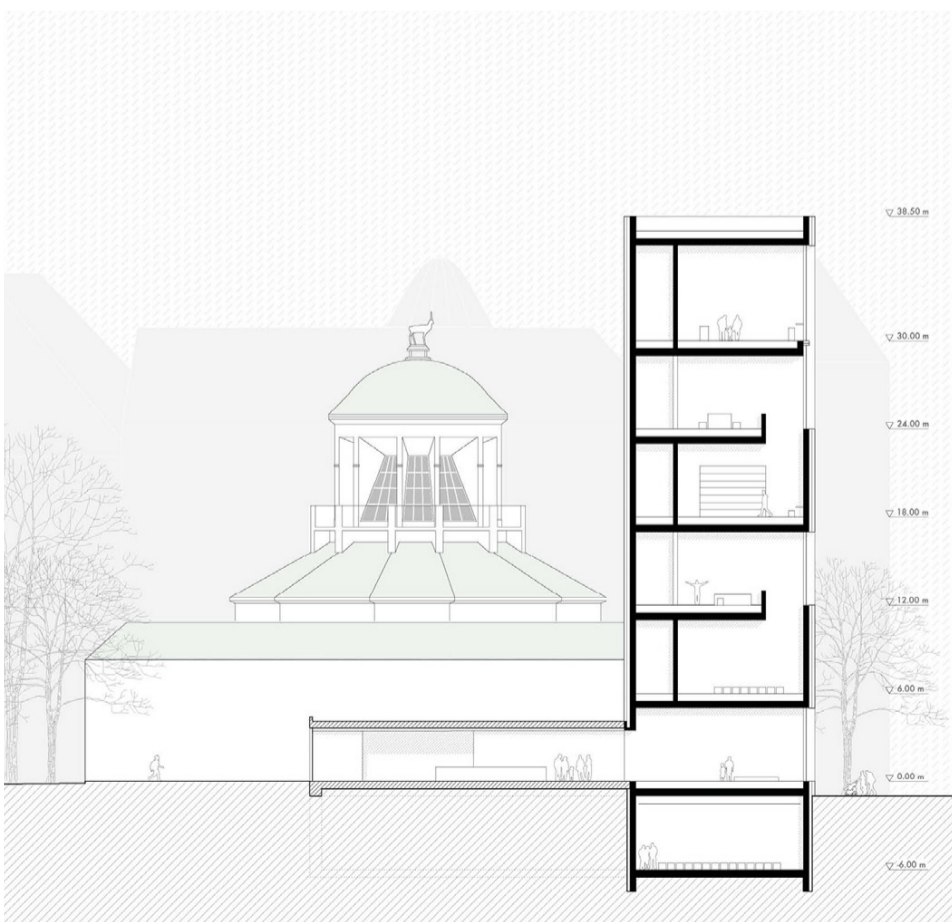
querschnitt
