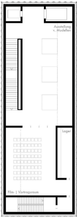
grundriss 1.og + 3.og
