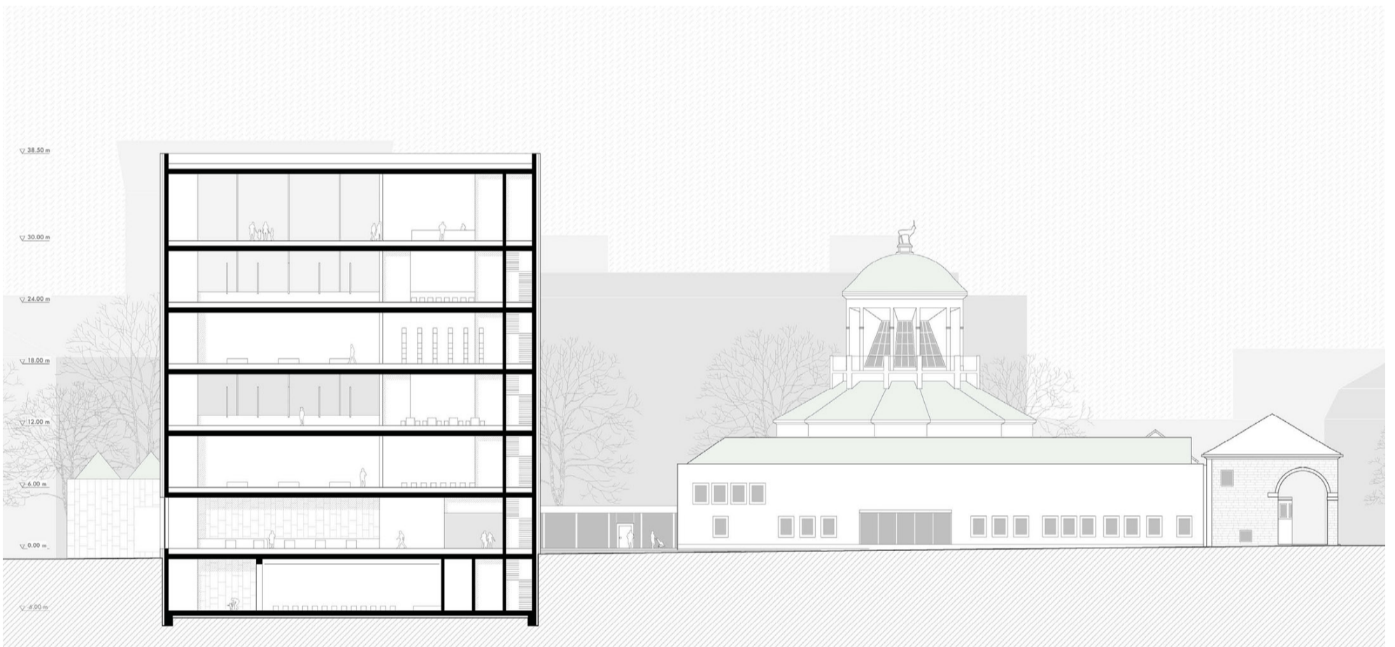
längsschnitt
