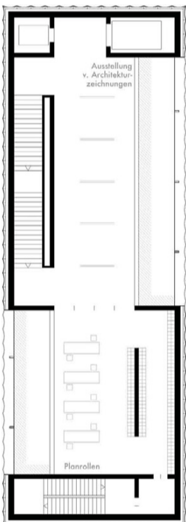
grundriss 2.og + 4.og
