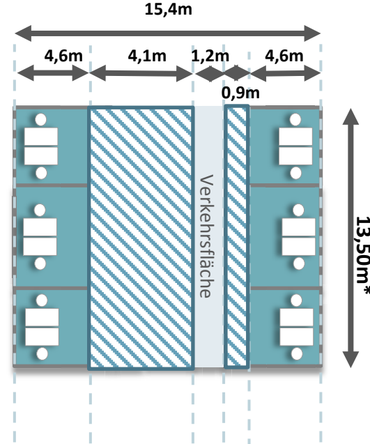
Bsp. 3 Kombibüro
