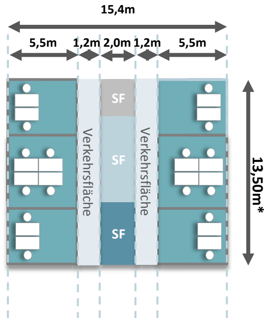
Bsp. 3 Kombibüro
