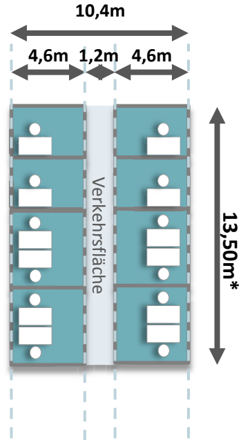
Bsp. 1 Zellenbürostruktur
